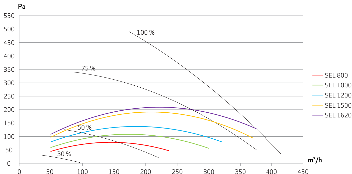
SEL-faktorer Combi Blueline - målt iht. EN13141-7 (Coarse/Coarse)
