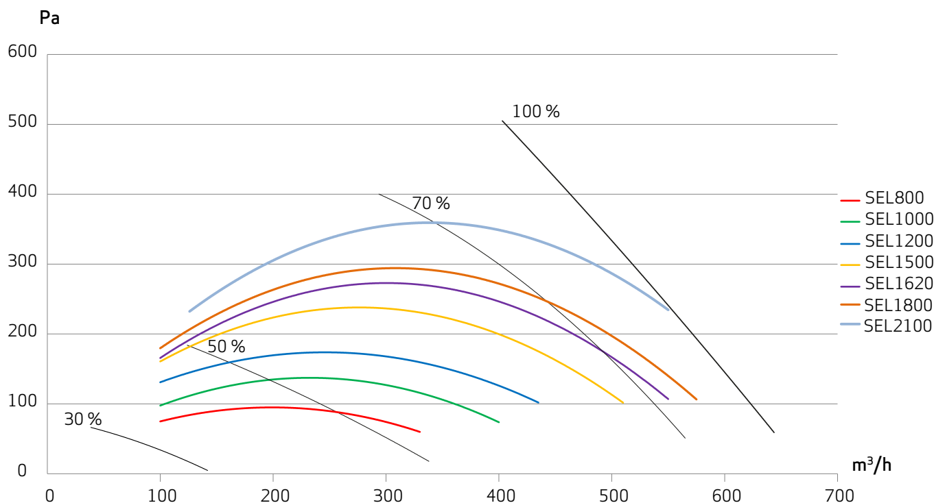
SEL-faktorer Premium Preheat 500 - målt iht. EN 13141-7 (Coarse/ePM1)
