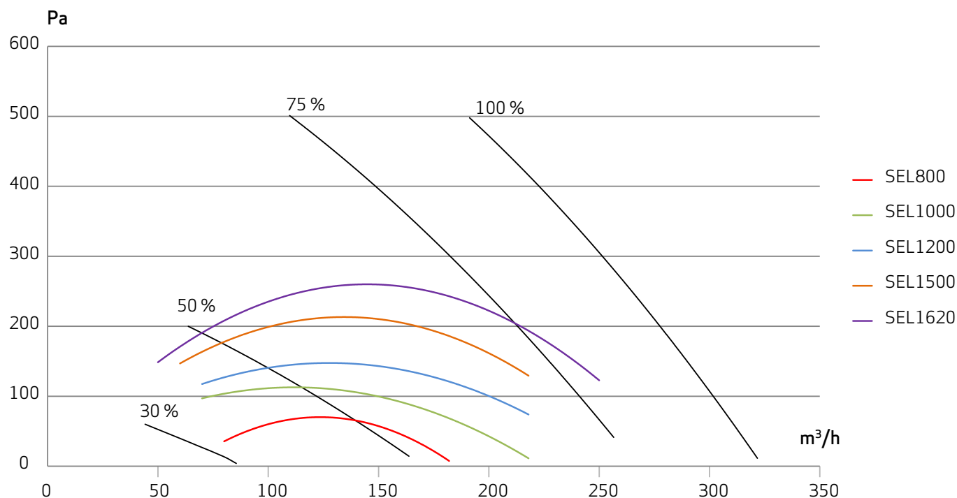
SEL-faktorer ECO 190 XL - målt iht. EN 308 (G4/G4:ALU)
