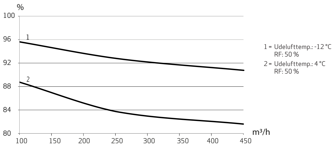
Temperaturvirkningsgrad iht. EN 308
