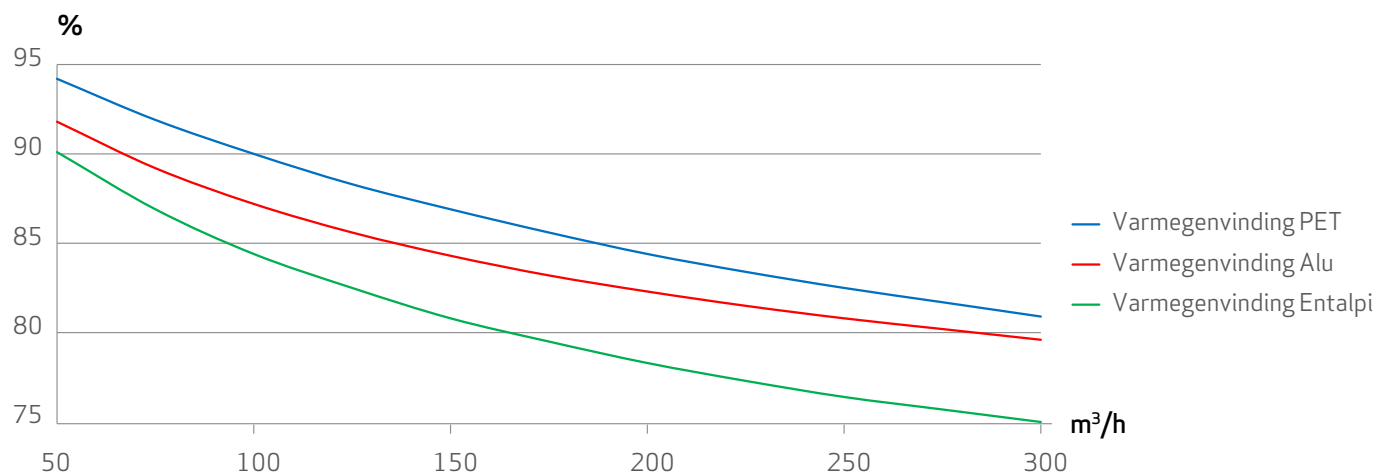
Temperaturvirkningsgrad iht. EN 308
