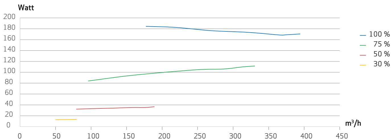
Effektøptag - for begge ventilatorer og styring
